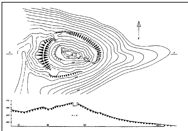
A Majorvár alaprajza
